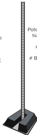
Base de béton hexagonale et poteau en "U" de 60" de haut # BBPOT 60 HEX Poids 225 lbs
